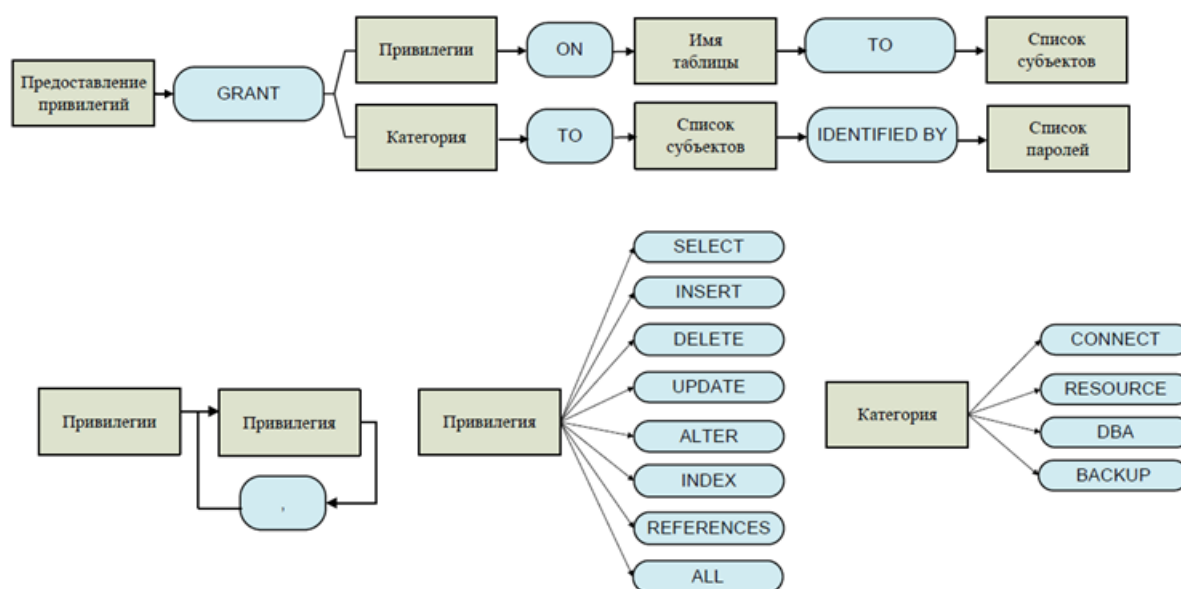
Рисунок 1. Схема оператора GRANT
