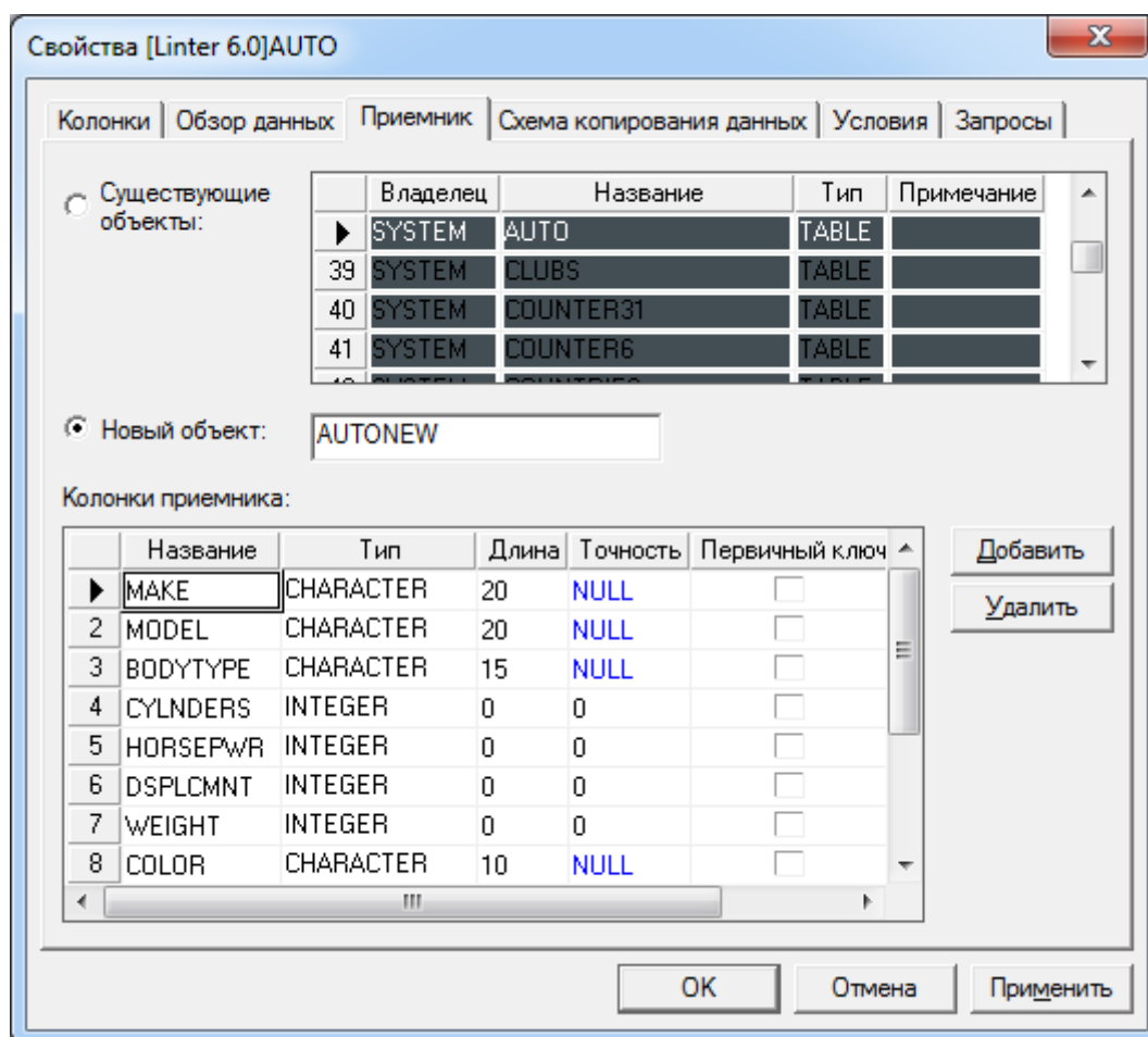
Рисунок 24. Свойства таблицы-приемника
