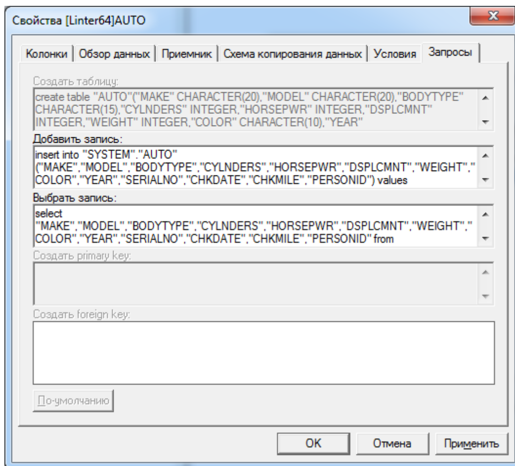
Рисунок 28. Текст SQL-запросов
