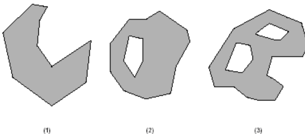
Рисунок 1. Примеры многоугольников
