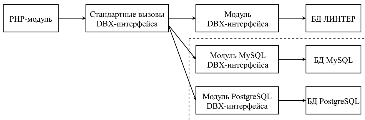
Рисунок 1. Схема взаимодействия PHP-модуля с СУБД
