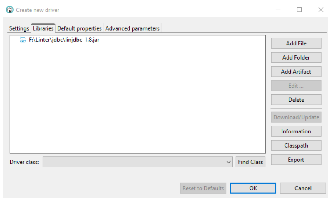
Рисунок 96. Параметры драйвера, вкладка Libraries, добавление драйвера
