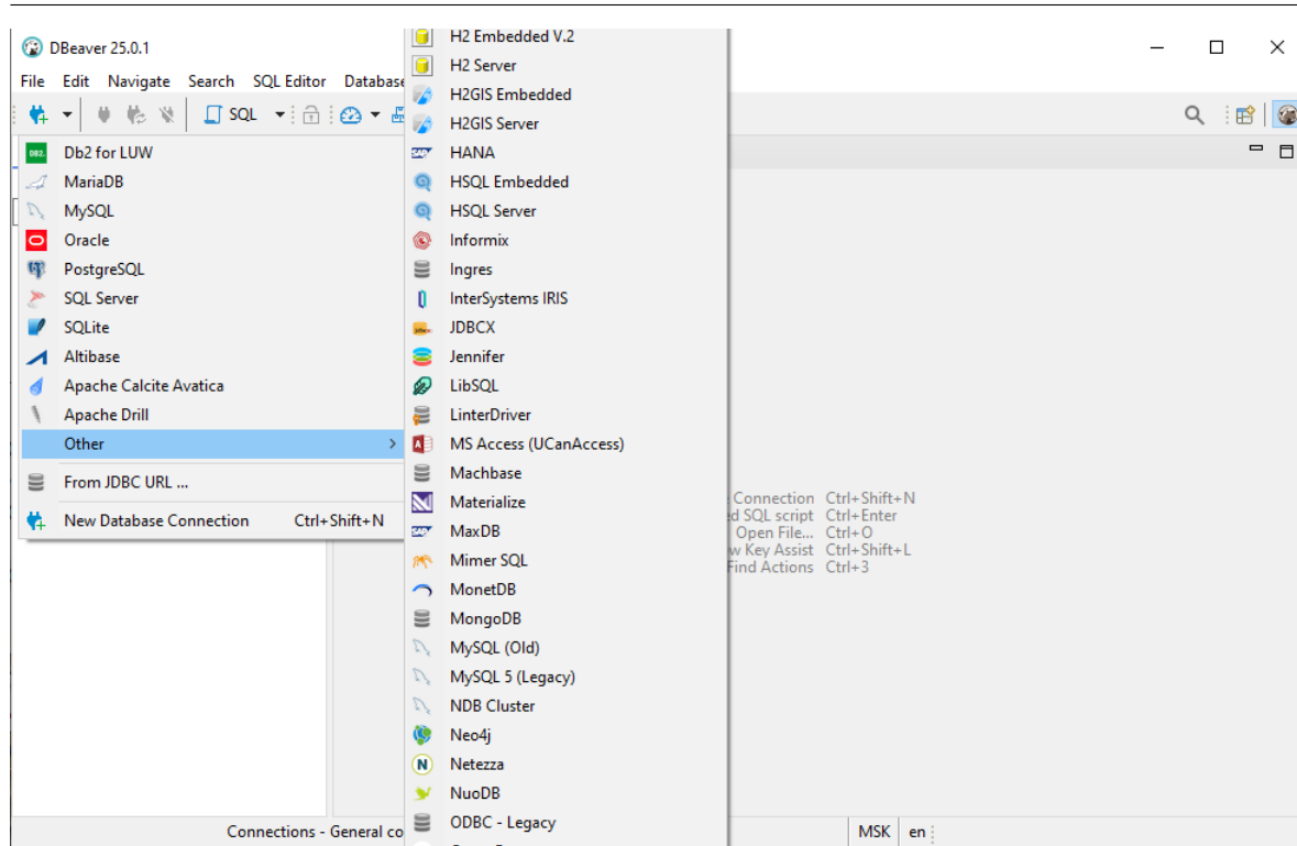
Рисунок 98. Добавление соединения
