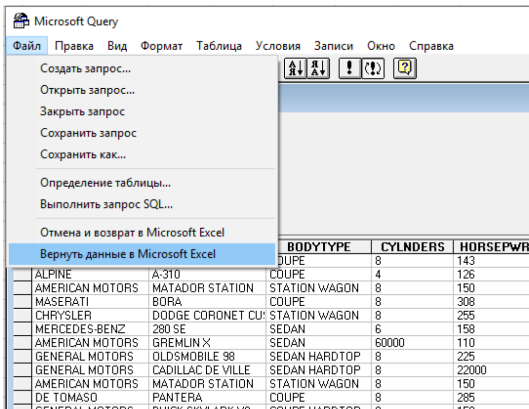
Рисунок 34. Вернуть данные
