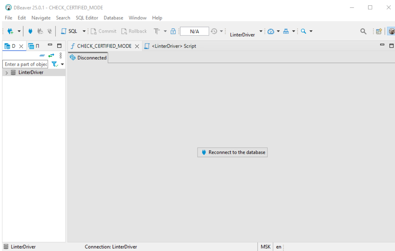
Рисунок 100. Список соединений
