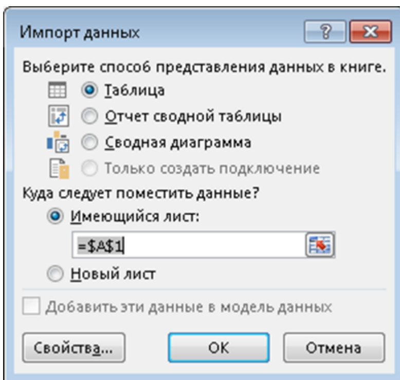
Рисунок 30. Импорт данных
