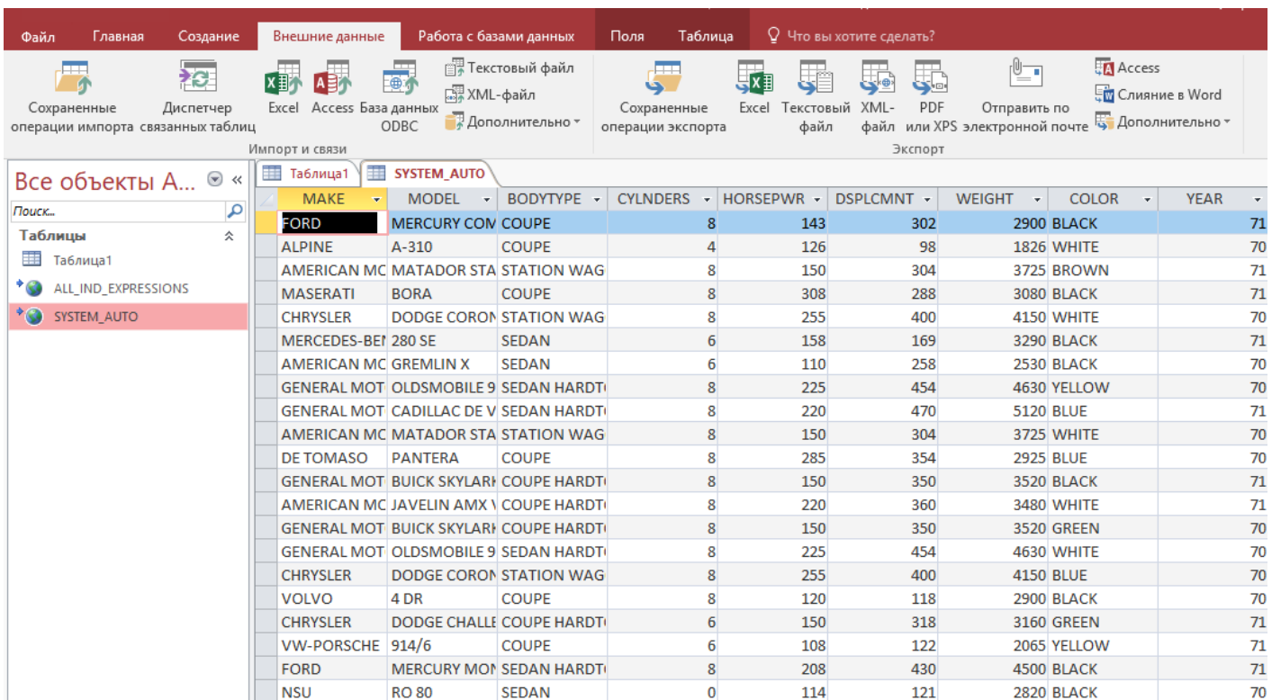
Рисунок 49. Результат подключения
