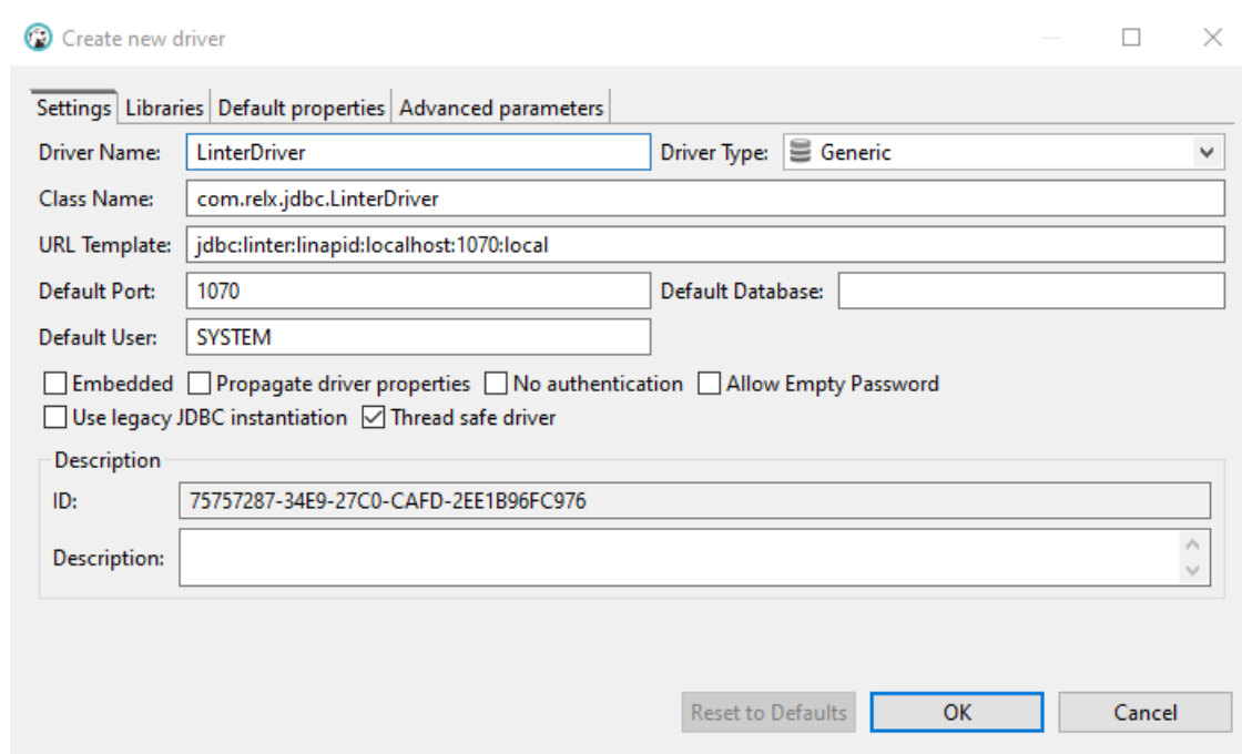
Рисунок 94. Параметры драйвера, вкладка Settings
