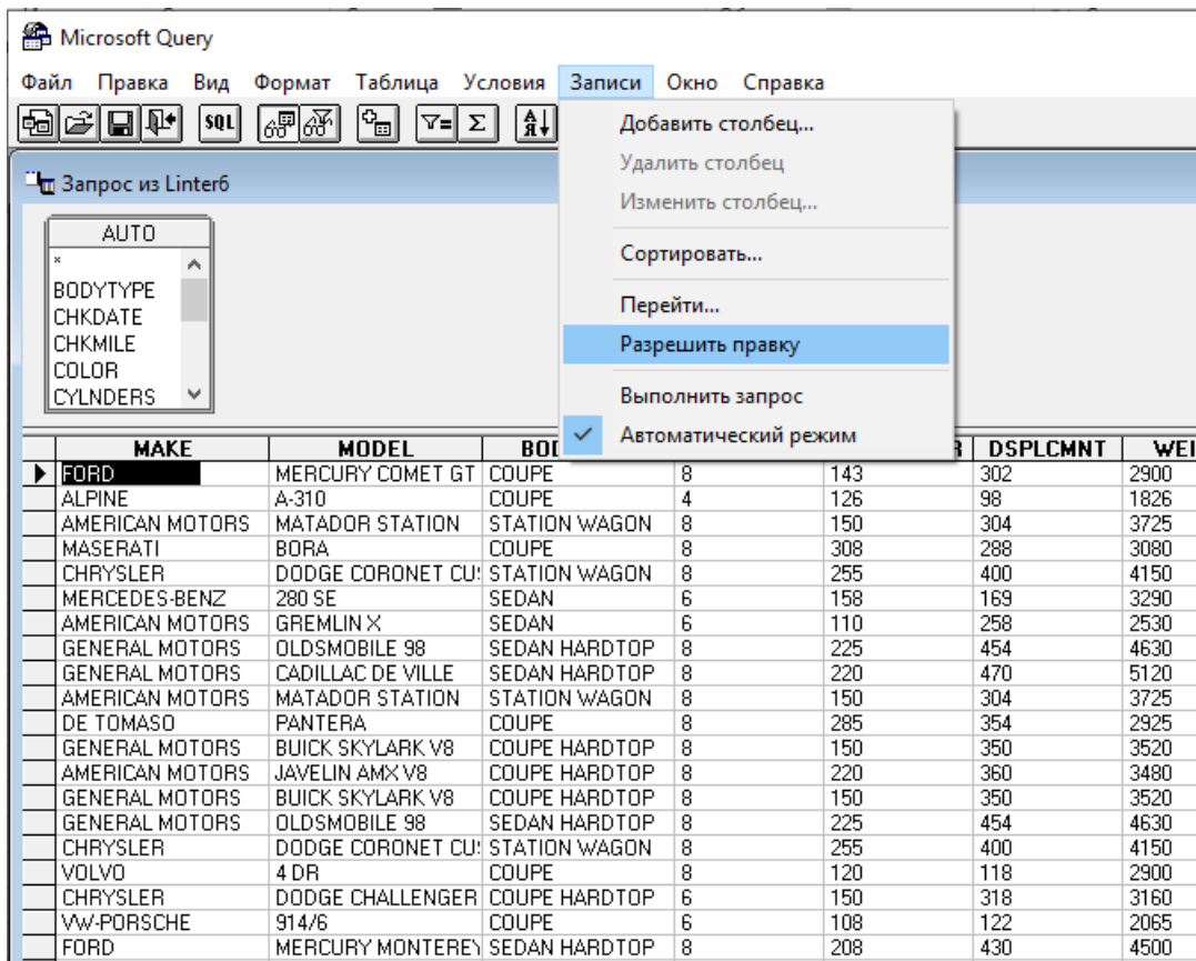
Рисунок 33. Разрешить правку
