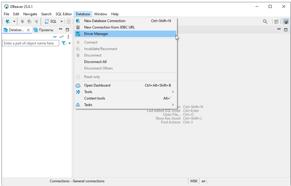
Рисунок 92. Выбор драйвера
