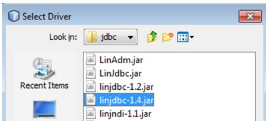
Рисунок 57. Выбор JDBC-драйвера
