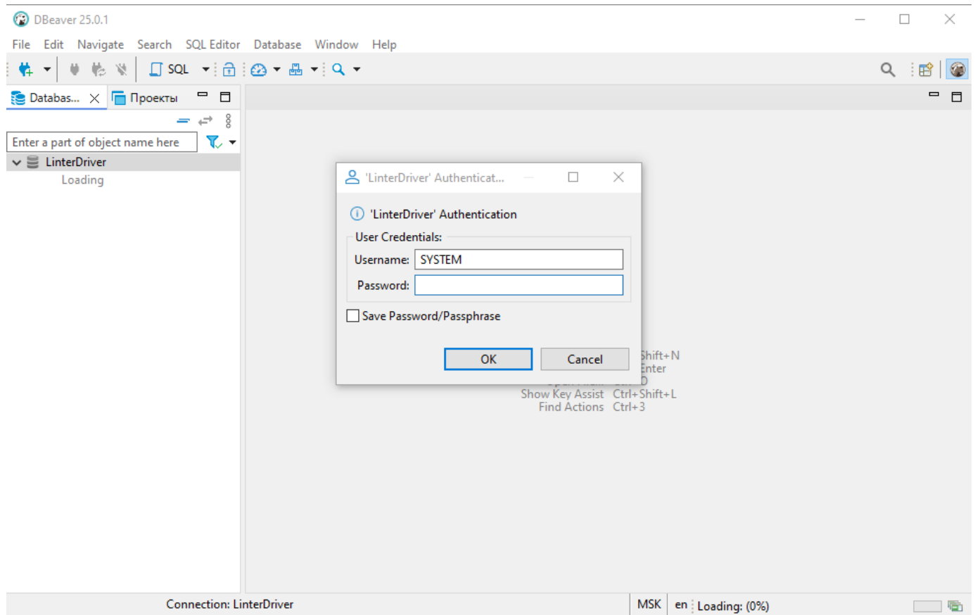
Рисунок 101. LinterDriver Authentication
