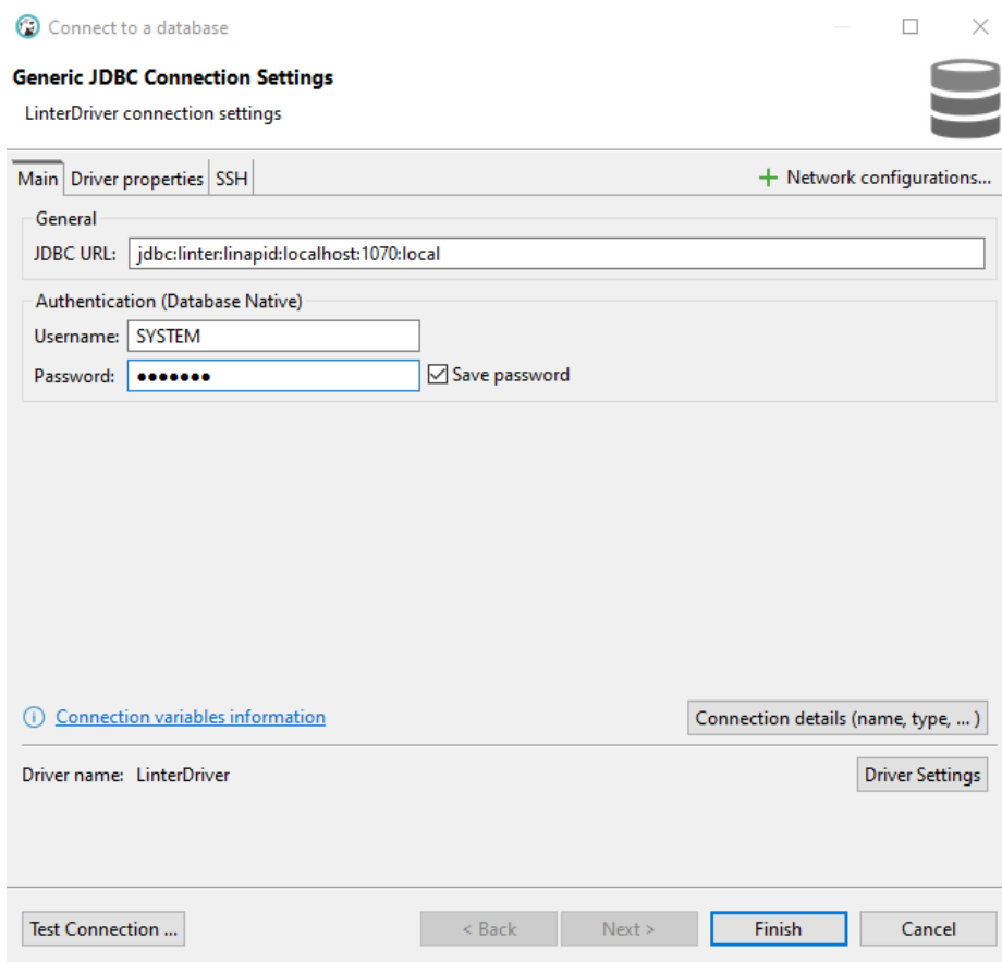
Рисунок 99. Параметры соединения
