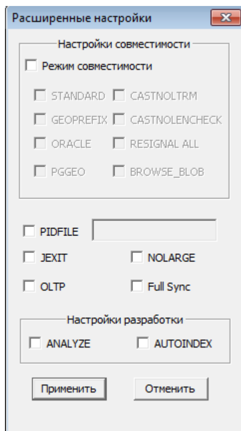
Рисунок 5. Расширенные настройки ядра
